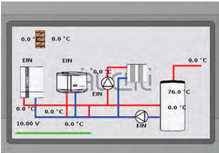
Steuerung einer kompakten Hybridanlage mit systemspezifischer Programmierung.
